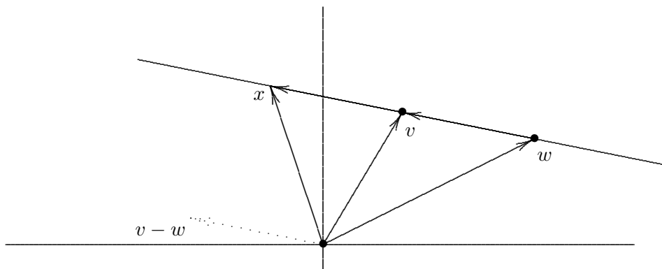
5.1. ábra: Egyenes a síkban
