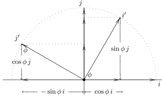
2.1. ábra: A sík forgatása
