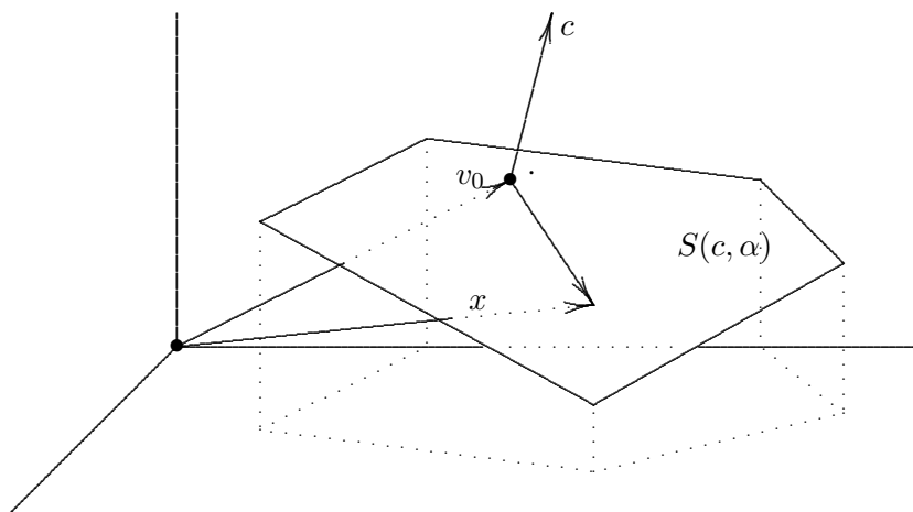
5.3. ábra: Sík a 3-dimenziós térben
