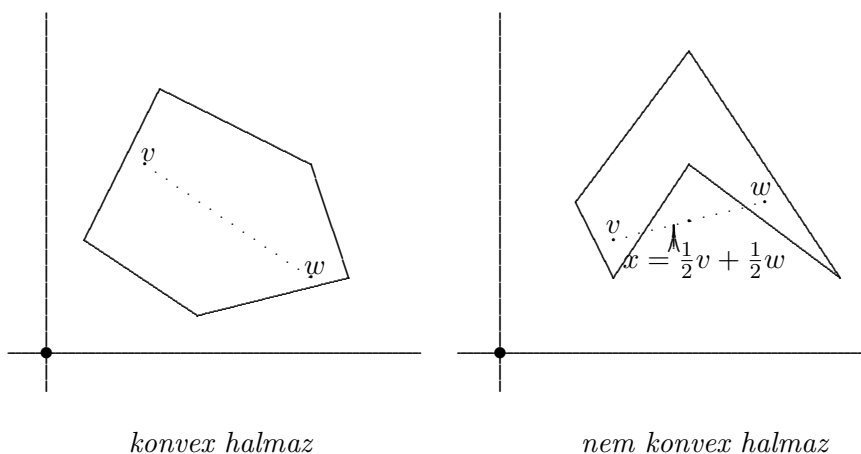
5.2. ábra: Konvex és nem konvex halmazok
