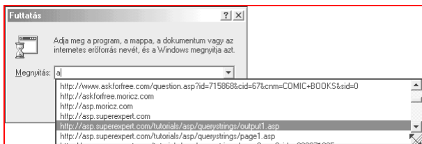
10. ábra. Automatikus kiegészítés egy átméretezhető tallózóval
