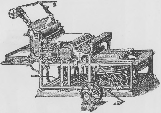
A bécsi Aner Alajosnak egyszerű gyorsajtóból tekerespapiros nyomtatására átszerkesztett egyszerű gyorsajtója 1860 tájáról.
