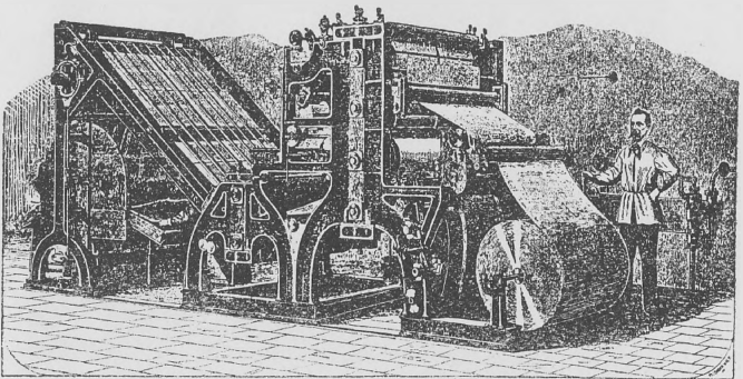
Walter-sajtó. A hatvanas évek vége felé használták a londoni „Times” nyomdájában. A tekerespapiros a gép jobb oldaláról kiindulva, gőzlő szerkezeten át jutott a nyomtatóműhöz. Ezt kétoldalas megnyomtatás után elhagyva, s a harántosan vágó hengerek közt széjjelszabdalódva, végül a kirakóasztalra került.
