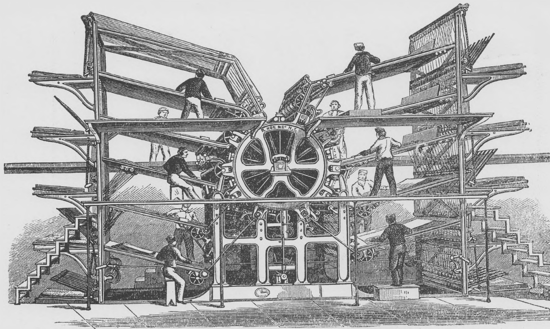
Hoe Robert 1847-ben épített „Mamut“ sajtója. A kétméteres átméretű henger fölületének egyrésze nyolc szedés- oldalnak kúpos záróeszközzel való rögzítésére, a többi része festékeldörzsölésre szolgált. Nyomóhenger tíz volt.
