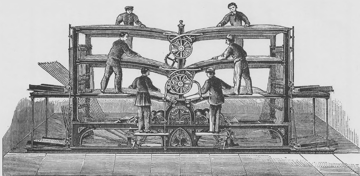
A párizsi Marinoni félkörös lemezekről nyomtató ujságsajtója 1869-ből. Amint látható: hat berakó munkás dolgozott rajta egyszerre. A nyomóhengerek fölváltva jobbfelé meg balfelé fordultak, s ezért „visszafelé is ható sajtó” (presse à réaction) volt a gép neve. 1870-re már tizenhat ilyen sajtó dolgozott Európa nagyobb ujságyomdáiban.
