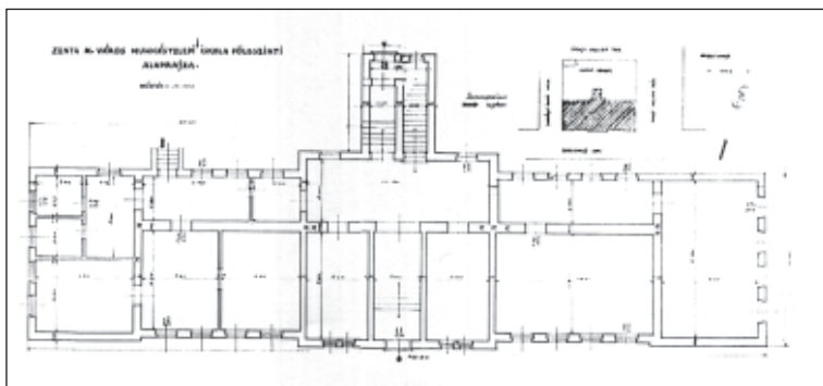
Az Eötvös-iskola alaprajza és helyszínrajza
