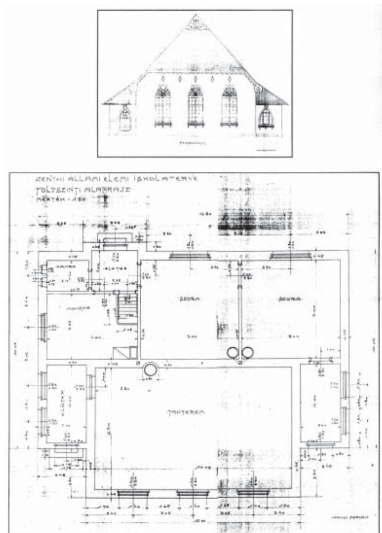
Az egy tantermes iskolák tervrajza (homlokzat, alaprajz)
