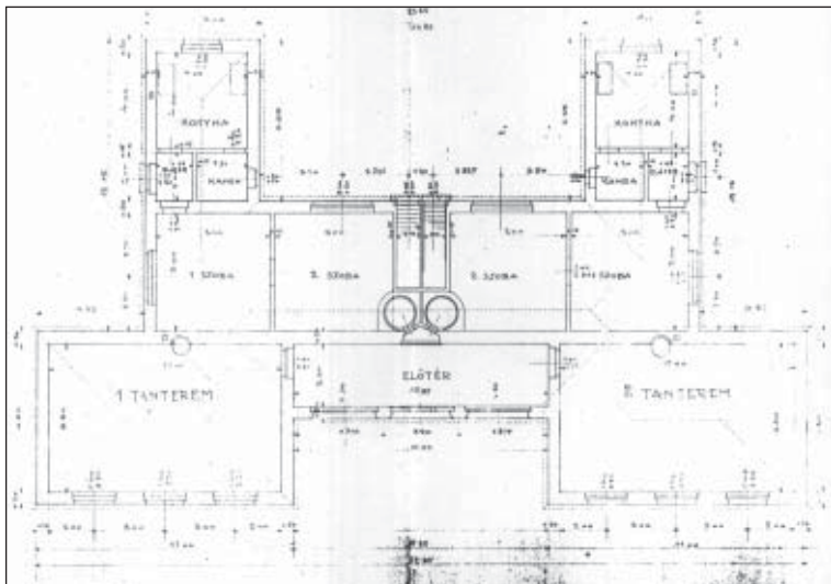
A két tantermes iskola tervrajza (alaprész)
