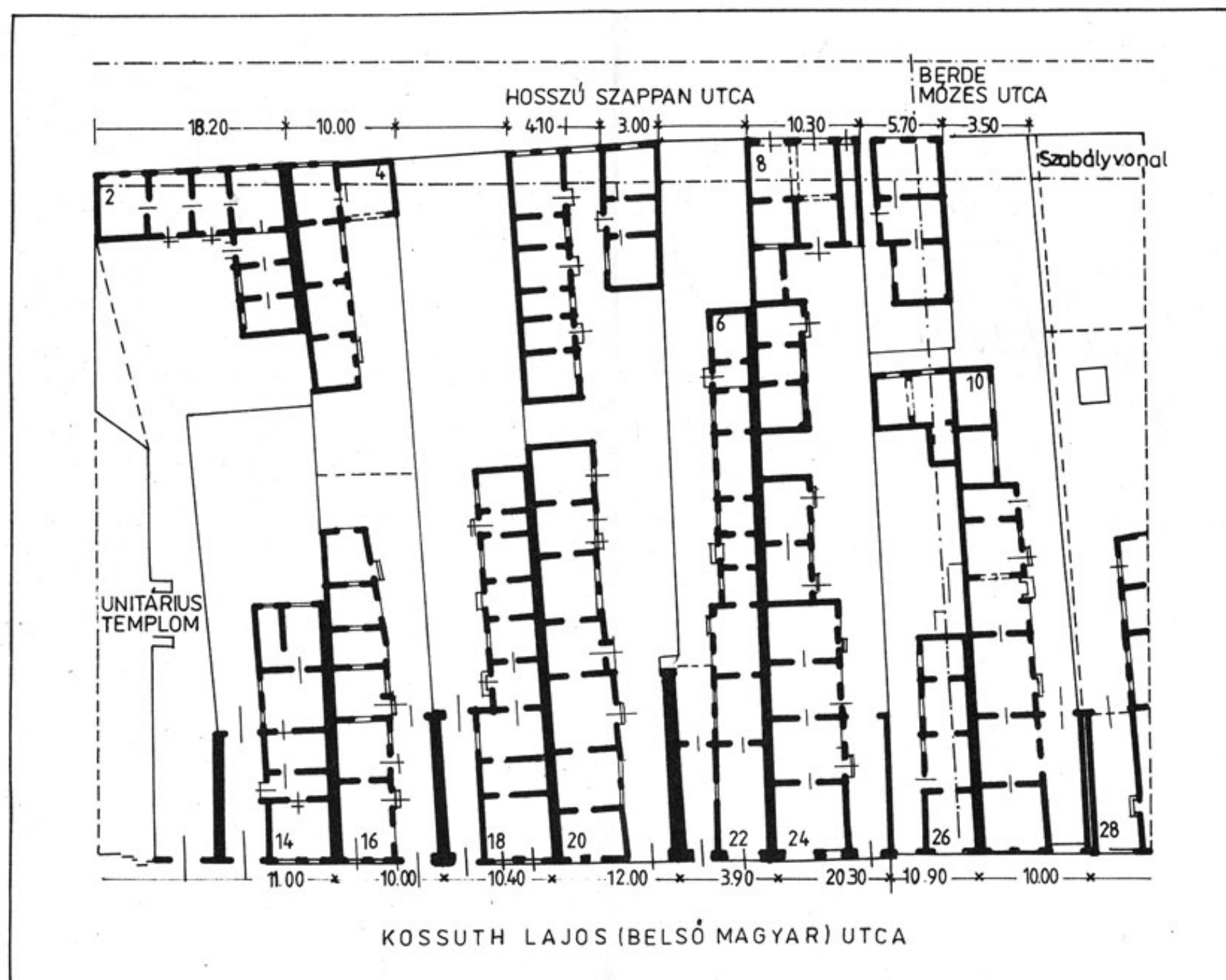
II. Az Unitárius Kollégium helyén lebontott épületek alaprajza Pákei Lajos 1899-ből származó felmérése alapján
