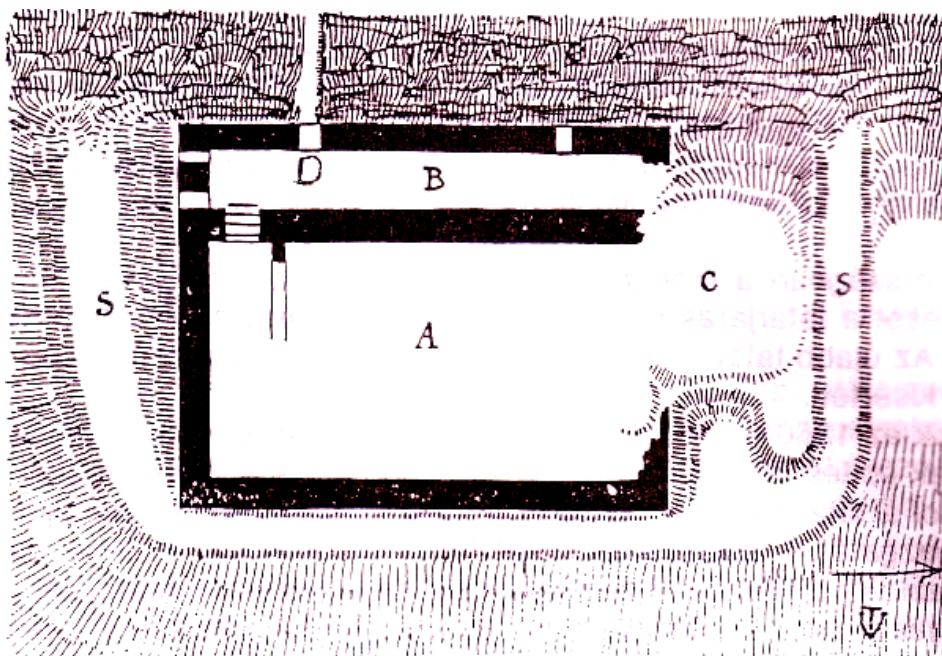
3. A MARKAZI VÁR ALAPRAJZA
