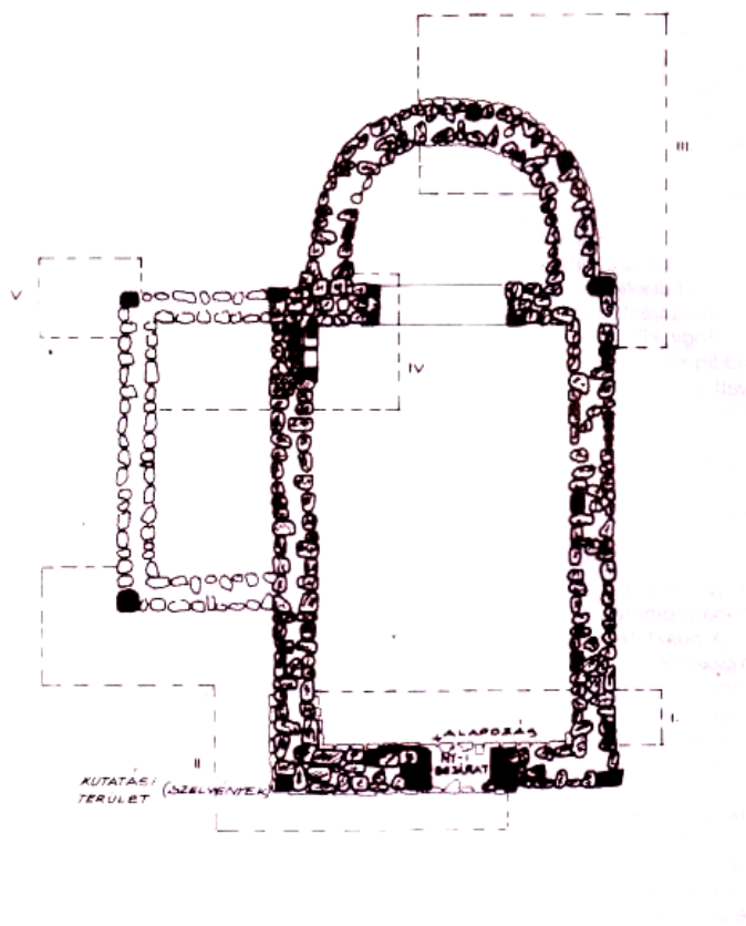
1. A markazi „pusztatemplom” alaprajza a kutatási szelvényekkel. A szaggatott vonalak jelzik az 1983-ban feltárt részeket, mely a templom területének mintegy negyedrésze.
