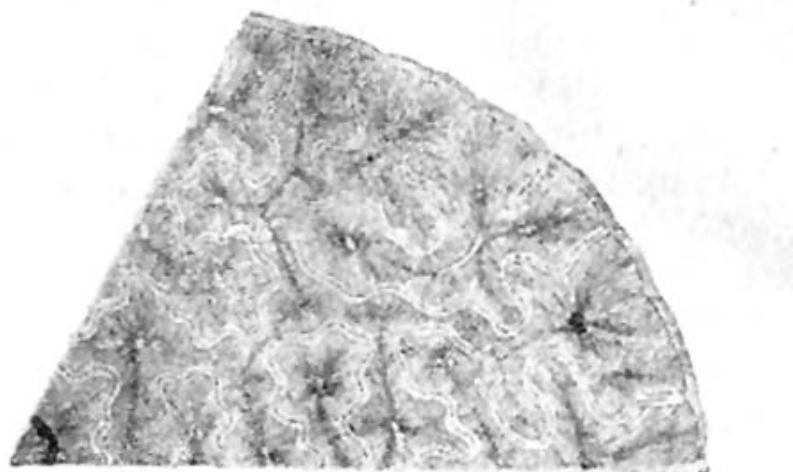
4. kép. Mastodonsaurus giganteus középső triászbeli ősszuszómászó kúpos fogának keresztmetszete. (A fogat különböző színű ásványi oldatok járták át s a fog különböző részletei más-más színűre festődtek.)
