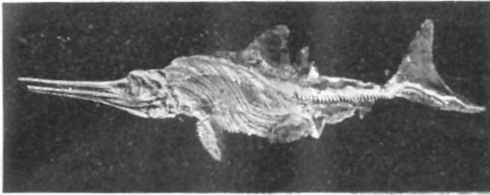
3. kép. Stenopterygius (Ichthyosaurus) quadriscissus QUENST. bőrrőstől megmaradt példánya a M. Kir. Földtani Intézet múzeumában. (A sötét színű uszonyrészekben a bőr tökéletesen megmaradt, helyenként 2 cm vastagságban).
