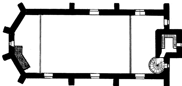
Pôdorys kalvínskeho kostola
