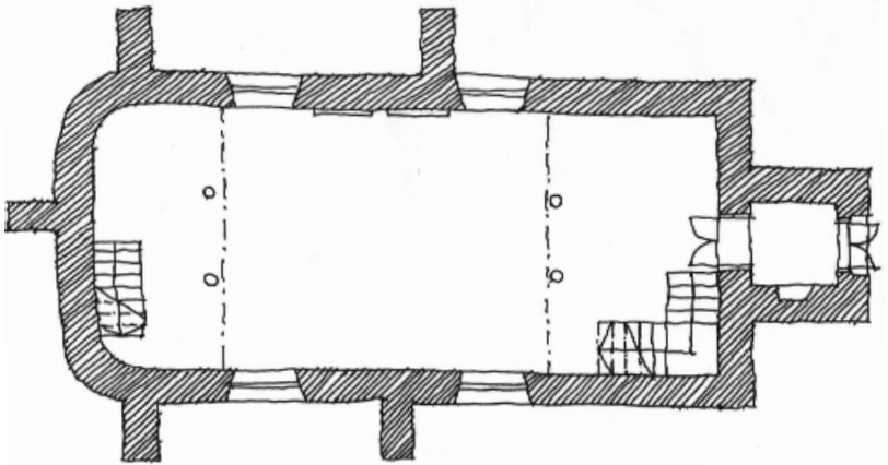
A templom alaprajza
