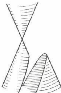
parabola
