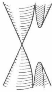
hiperbola
