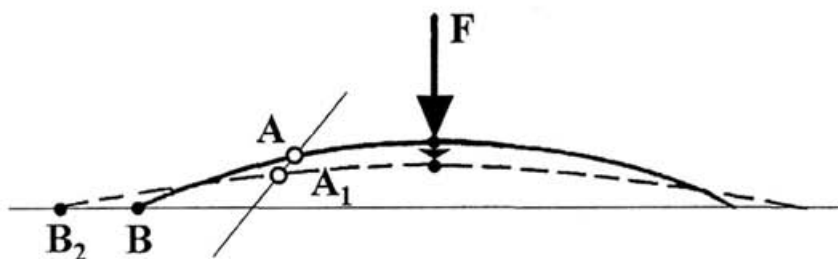
64. ábra Íves tengelyű tartó elmozdulása terhelés hatására
