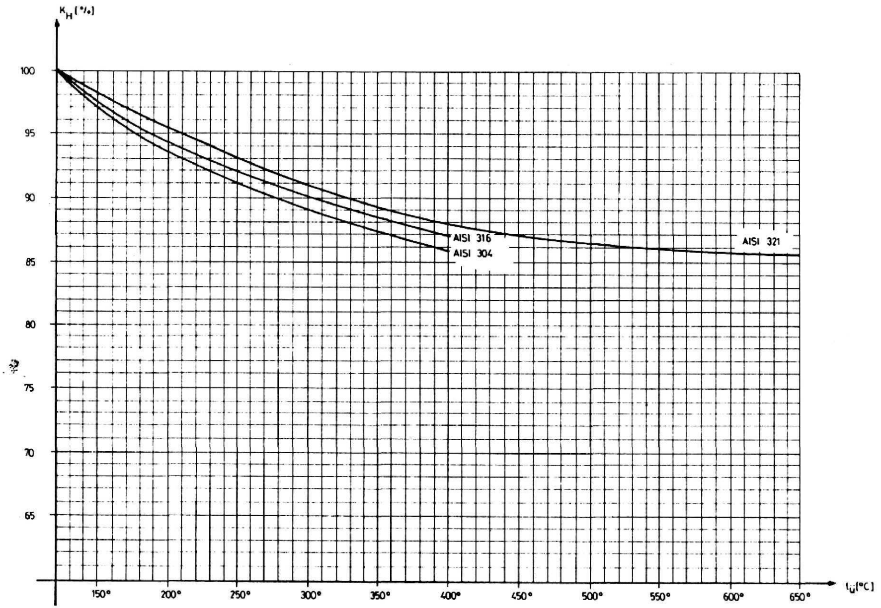
6. diagram Diagram a K_H löketkorrekciós tényező meghatározásához az üzemi hőmérséklet függvényében
