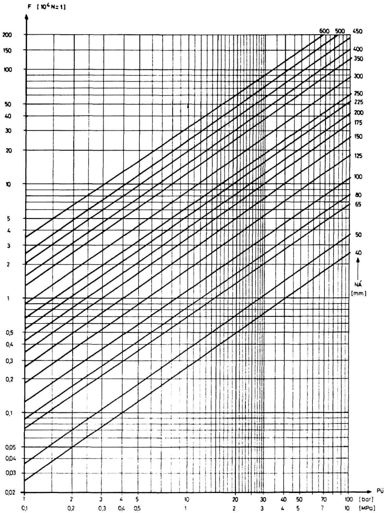
7. diagram Axiál kompenzátorok reakcióereje a névleges átmérő és az üzemi nyomás függvényében
