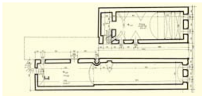
Emeleti, földszinti és pince alaprajz
