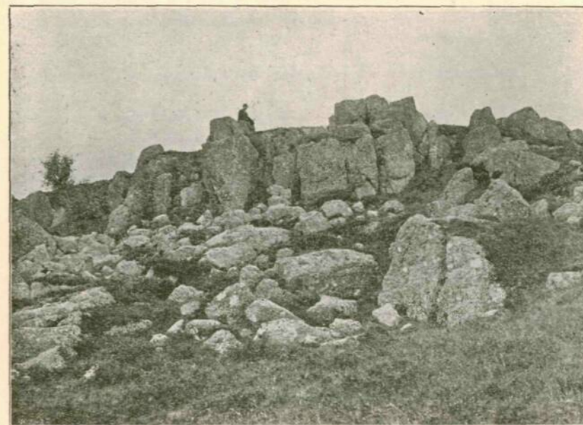
3. ábra. Krétakorú konglomerátum-sziklák a Botesi hegytetőn 1200 m t. f. magasságban.
