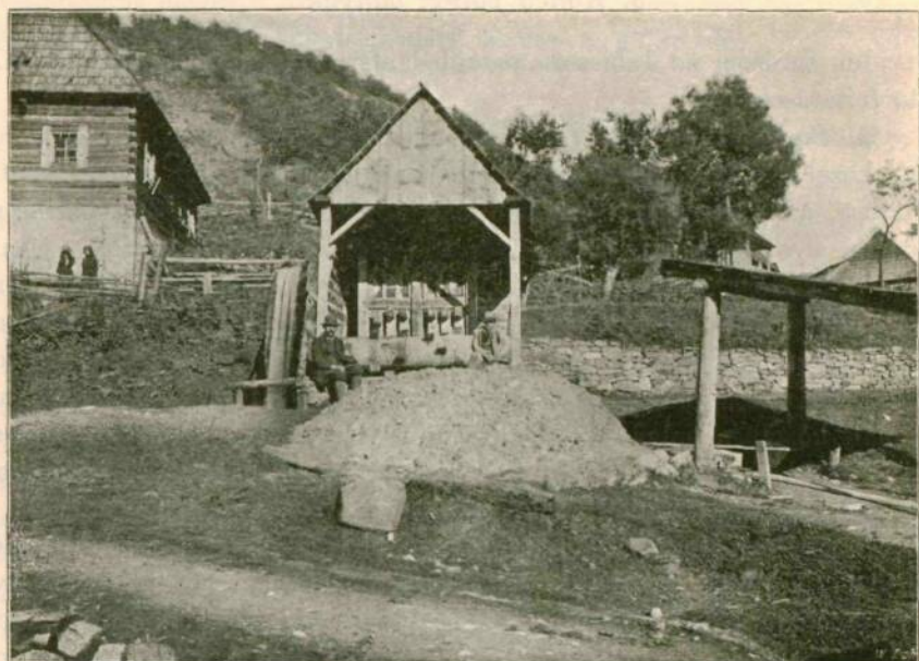
10. ábra. Hatnyilas aranyzúzómalom a bucsúmiszbitai templommal szemben.
