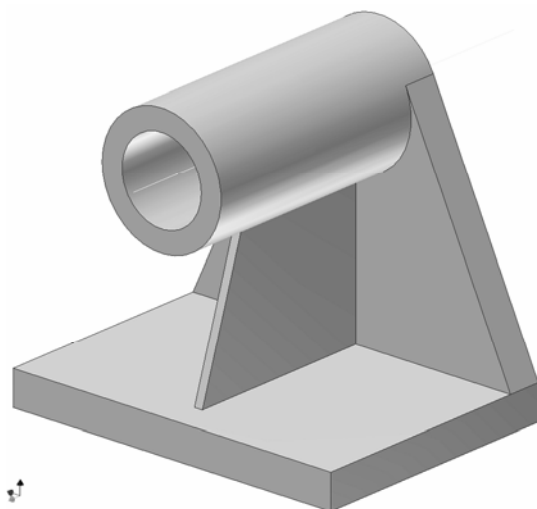
2.63. ábra A borda sajátosság első változata
