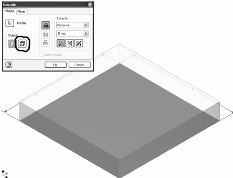
2.27. ábra Az első Extrude művelet
