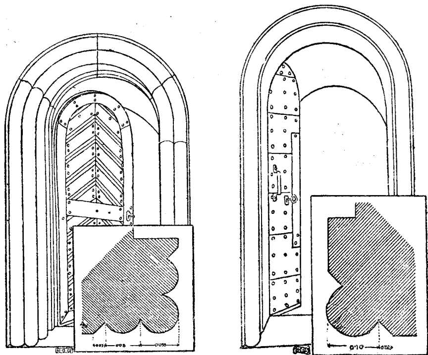
5. és 6. A csiksomlyói Szent Péter plébániatemplom ajtókeretei.
