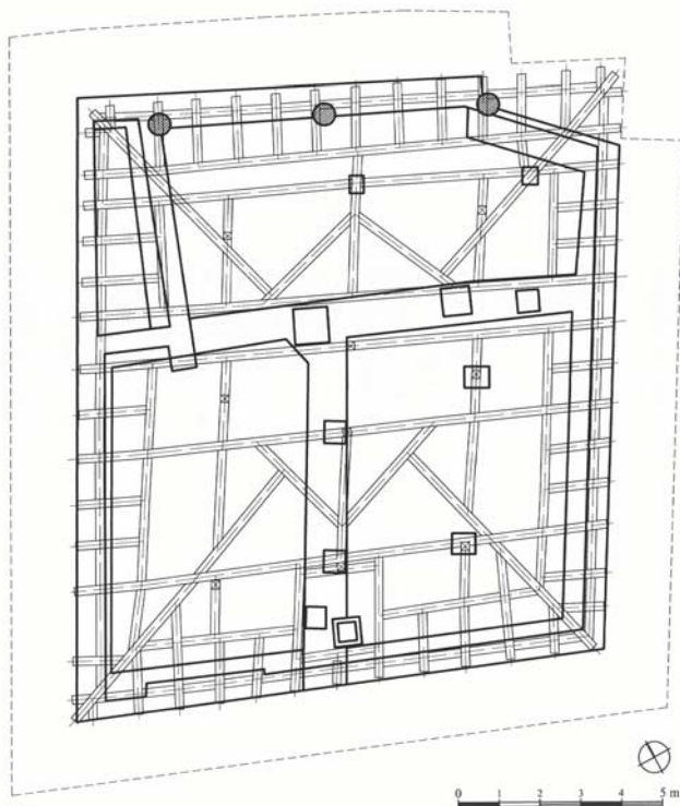
24. A Veres-bástya padlásának alaprajza.
