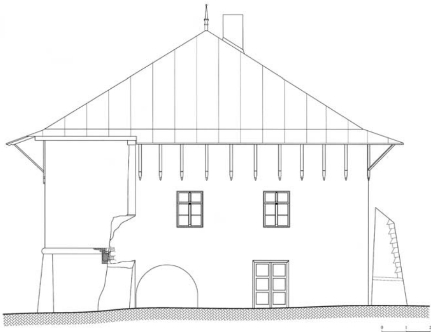
12. Északkeleti homlokzat.
