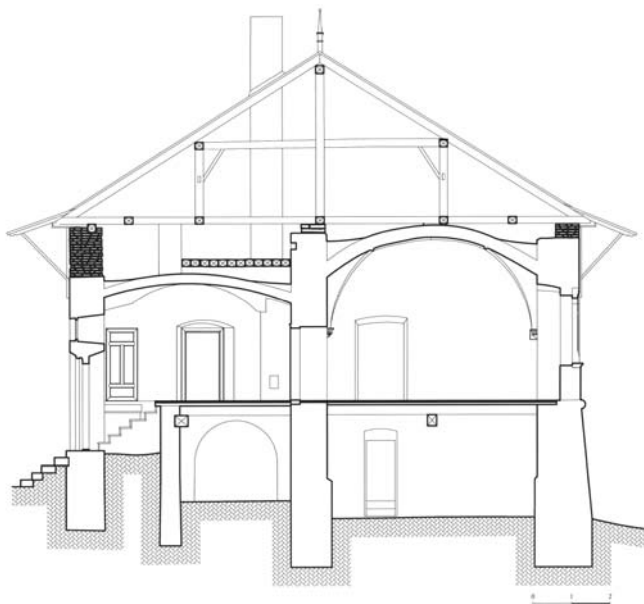
25. Keresztmetszet.
