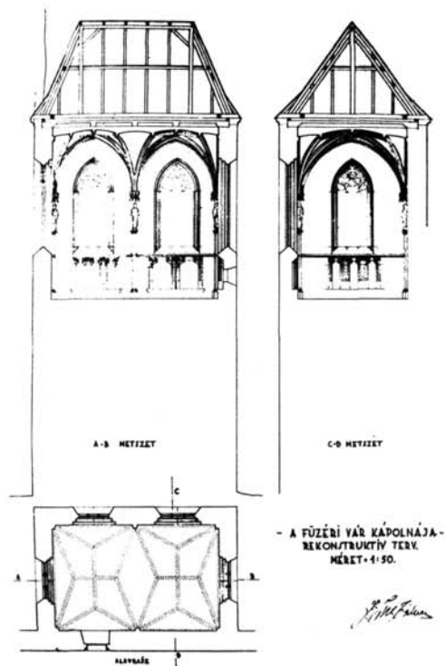
25. kép. A kápolna rekonstrukciós terve, Lux Kálmán, 1935. Belső. OMF (reprodukció Hász András)
