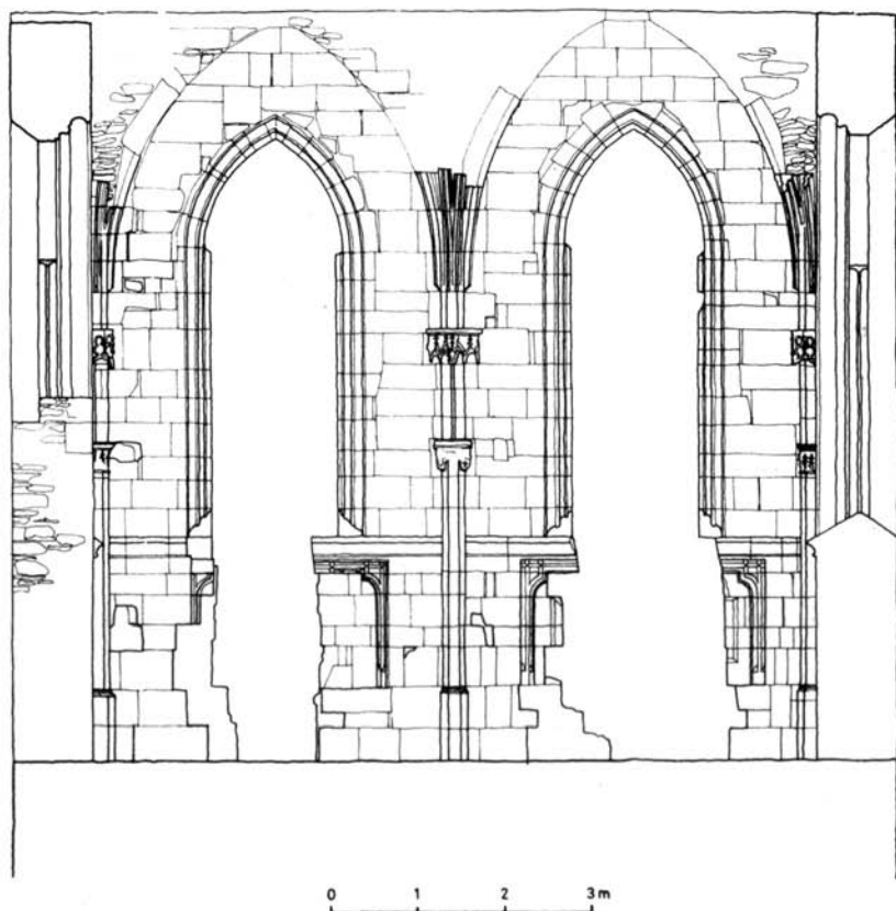
28. kép. A kápolna déli belső homlokzatának felmérése, 1979. (Teleki Katalin rajza)
