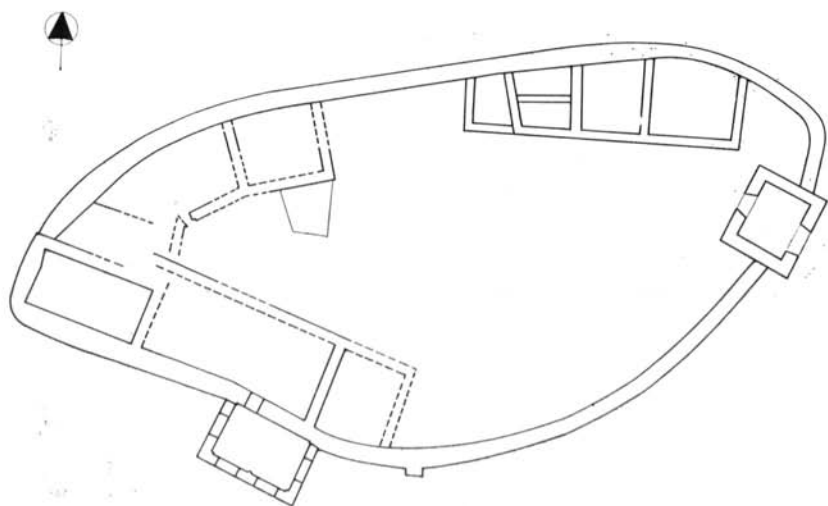
30. kép. A 14—15. századi vár alaprajza az eddigi kutatások alapján (László Csaba rajza)
