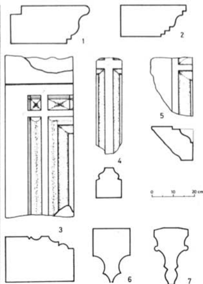
32. kép. Gótikus és reneszánsz kőfaragványok a várból (László Csaba rajza)
