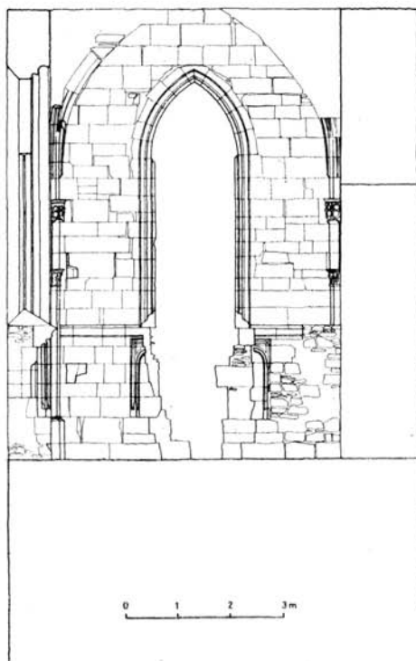
29. kép. A kápolna nyugati belső homlokzatának felmérése, 1979. (Teleki Katalin rajza)
