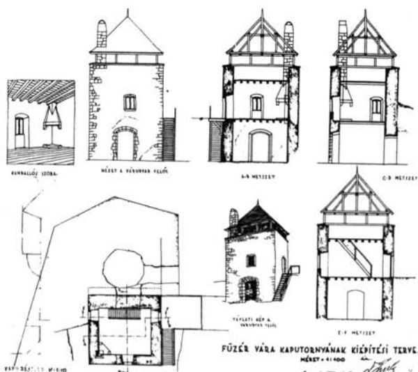
63. kép. A kaputorony kiépítésének terve, Lux Géza, 1935. OMF (reprodukció Hász András)
