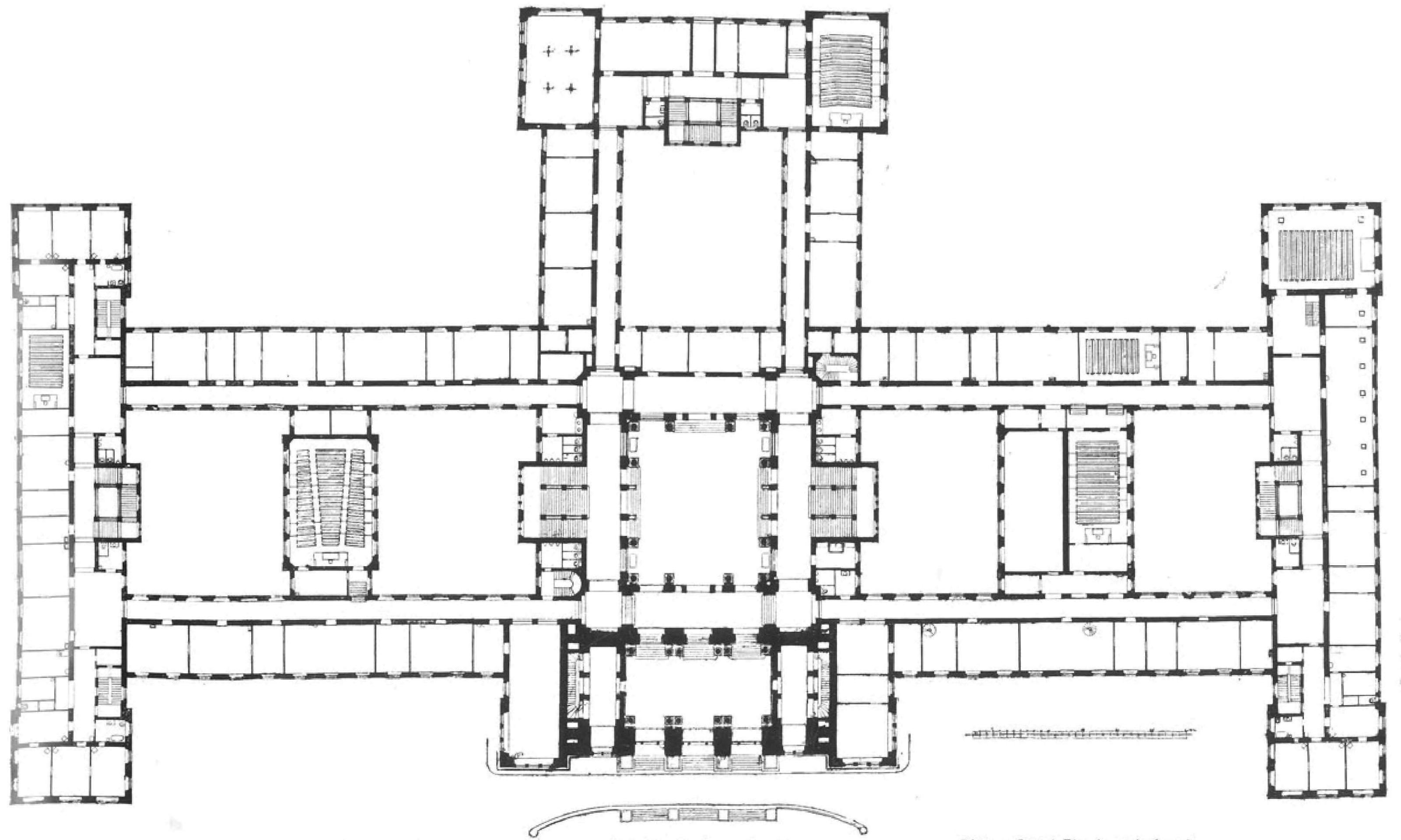
Központi épület. Földszinti alaprajz
