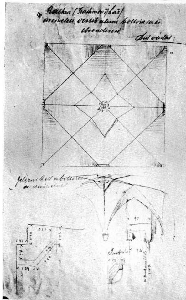
12. A Wolphard–Kakas-ház vestibulumának boltozata
