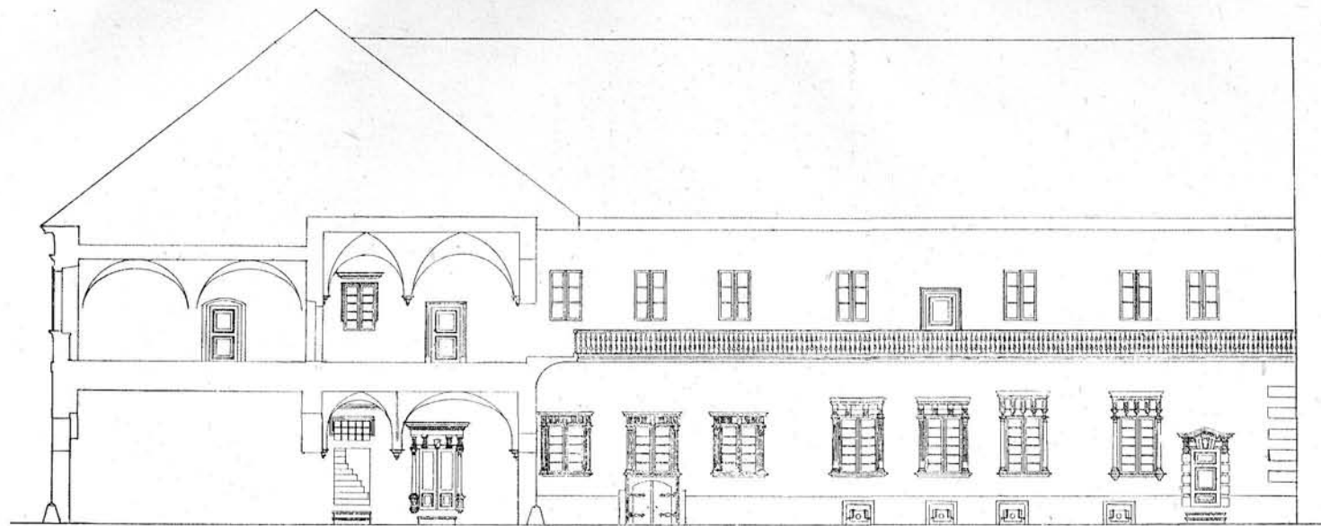
8. A Wolphard –Kakas-ház hosszmetsete
