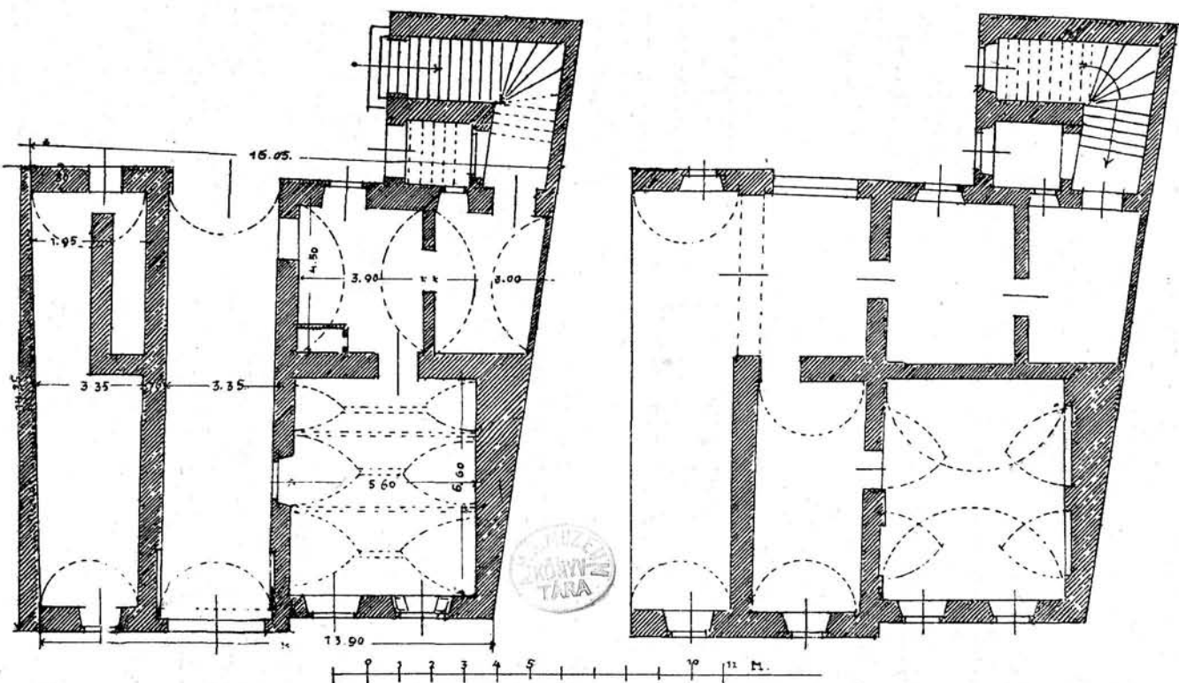
23. Az óvári u. n. Basta-ház a Karolina-ter déli során. Földszinti (baloldalt) és emeleti (jobbaldalt) alaprajz
