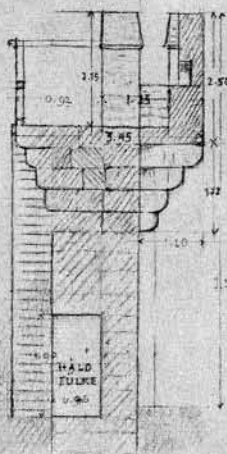
AZ ÖRFÜLKE KERESZT AB METSZETE.
