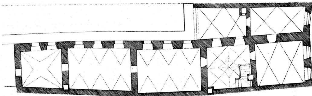
15. A Wolphard-Kakas-ház emeleti alaprajza
