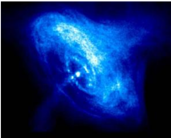
32. ábra (neutroncsillag)
