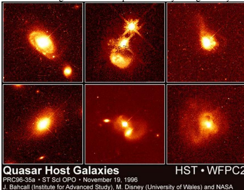
46. ábra (kvazárok)
