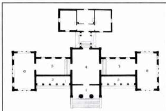
5. kép. A kibővített Aquincumi Múzeum alaprajza. 1896. 1-3: kőemlékek, 4: kő- és bronzszobrok, sírleletek, 5: kőemlékek, 6: építészeti maradványok, 7: kőemlékek, 8: a kézművesipar termékei, érmek.
