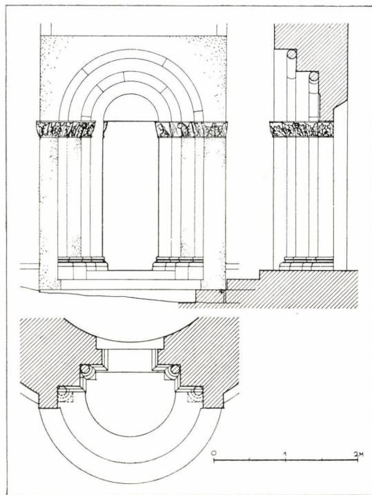
A Szent Mihály-kápolna kapujának műszaki rajza Lux Géza műegyetemi adjunktustól.
