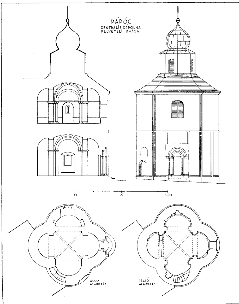
Lux Géza műegytemi adjunktus rajza.
