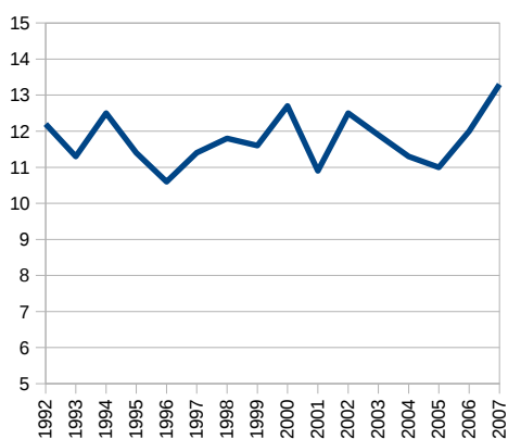
Felszíni éves középhőmérséklet Budapesten, °C
