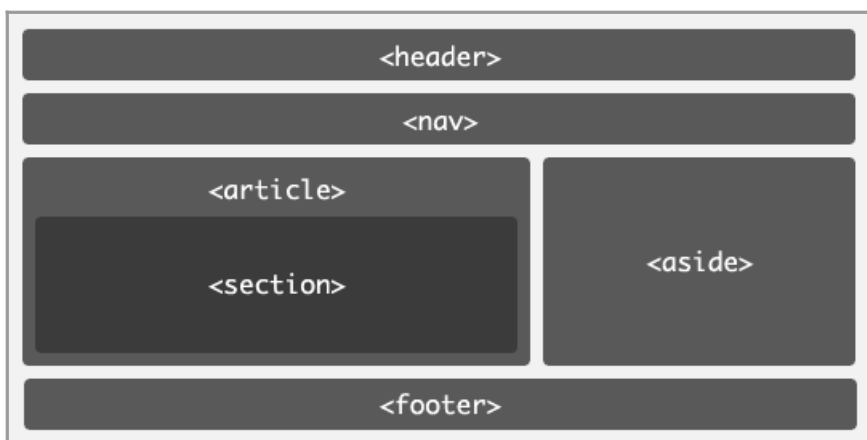
31. ábra. A div elemek helyett header, nav, section, article, aside és footer
