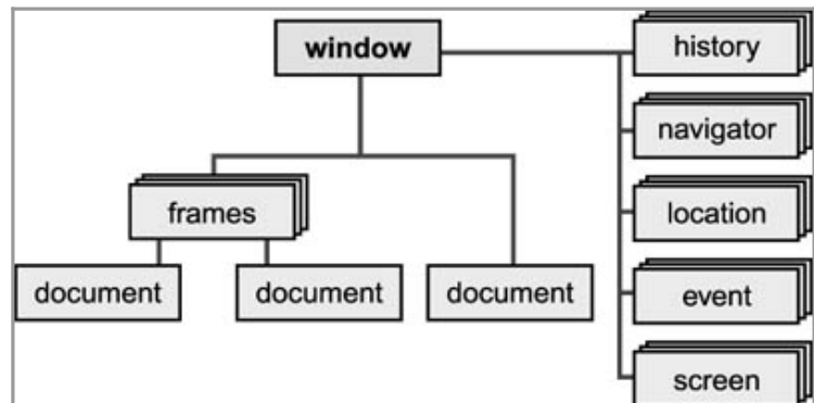
74. ábra. JavaScript objektumhierarchia
