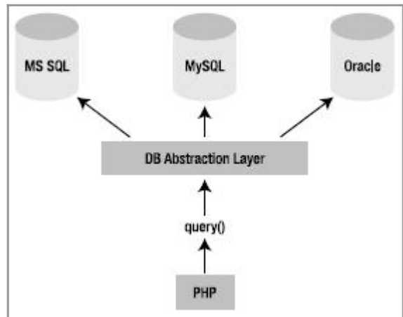
55. ábra. Adatbázis absztrakciós réteg
