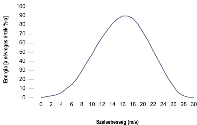
28. ábra: ekvivalens regionális energiagörbe
