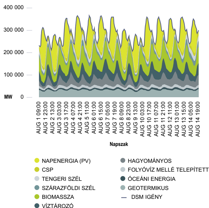
42. ábra: az energiatermelés (MW-ban) különböző energiaforrásokról, és az európai összesített igény a 2003. augusztusi szélsőséges helyzet alatt
