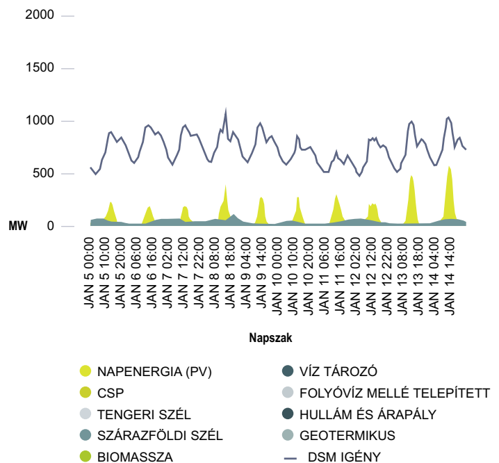
42. ábra: az energiatermelés (MW-ban) különböző energiaforrások felhasználásával, és a helyi igény az 1997. januári szélsőséges helyzetben, Hollandiában. ez a helyszín a szélsőséges időszak alatt végig energiainportra szorul
