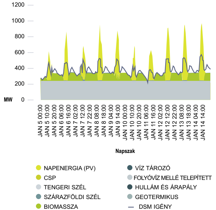
44. ábra: az energiatermelés (MW-ban) különböző energiaforrások felhasználásával, és a helyi igény az 1997. januári szélsőséges helyzetben, Dél-Németország egy másik részén. van olyan időszak, amikor többlettermelés tapasztalható, és előfordul, hogy nincs elegendő energia
