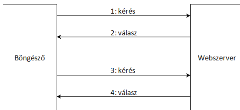
6. ábra - A HTTP kérések és válaszok
