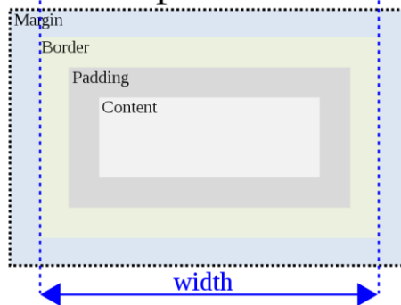
27. ábra: IE és W3C doboz modell (Forrás: Wikipedia)
