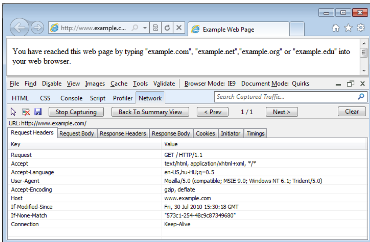
7. ábra – Az Internet Explorer 9 Developer Toolbar Network fülén a forgalom minden részlete látható
