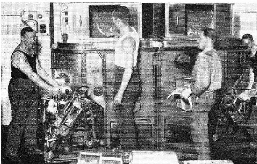
Iker-öntőgép rotációslemezek részére Termelése percenként négy ujságoldal
