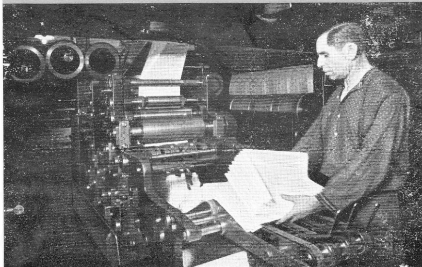
A Hungária Nyomda rotációs gépein készült az Esti Kurir, a Mai Nap, a Reggeli Újság, a Rádió Újság és még számos más heti lap
