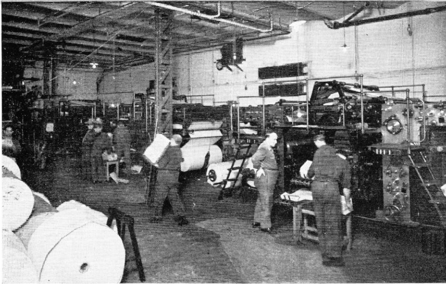
Rotációs gépterem: egy 48 oldalas és három 32 oldalas rotációs gép
