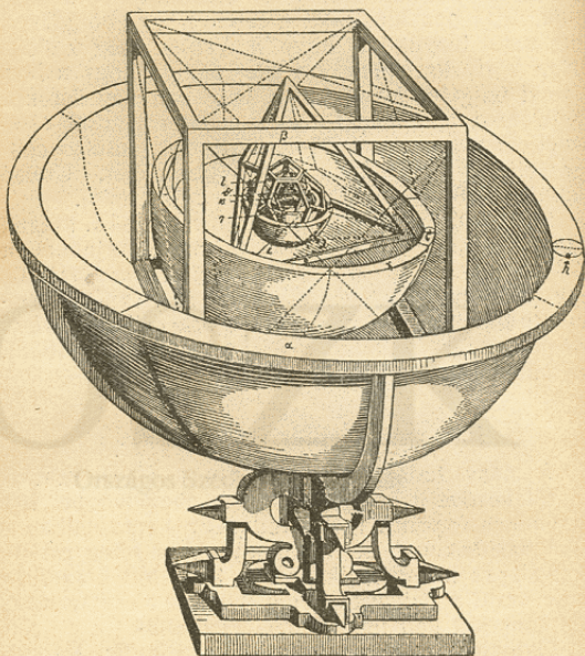
Kepler bolygórendszere.
