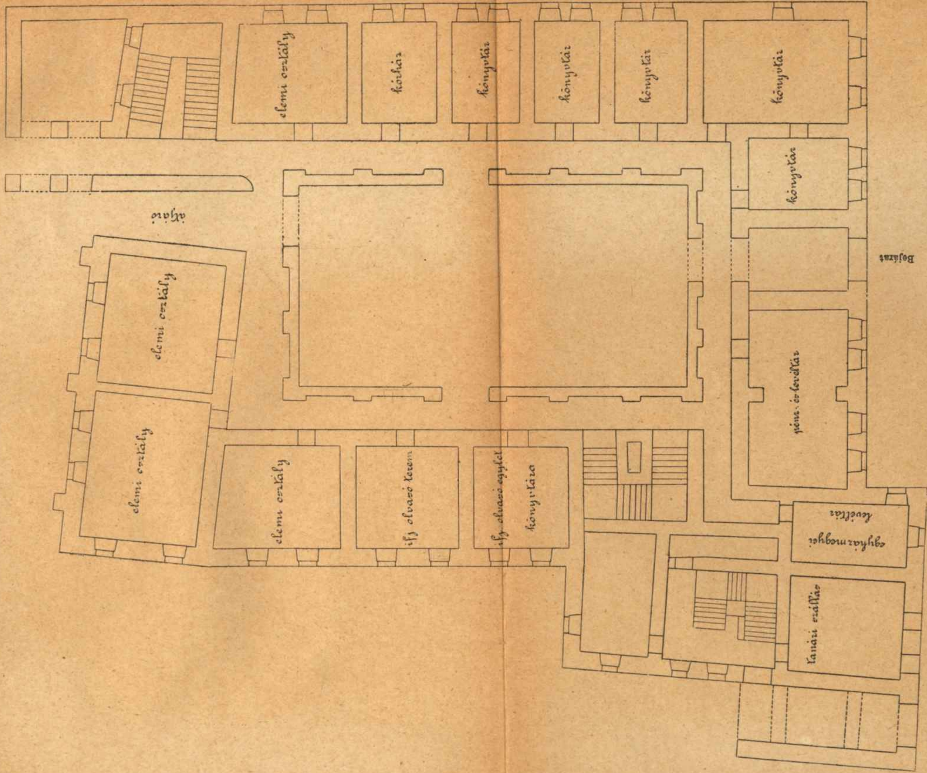
FÖLDSZINT.
