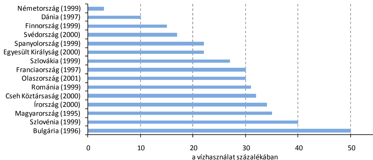
19. ábra: A közösségi vízhálózatok veszteségének mértéke (xx)
