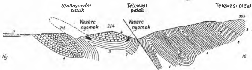
3. ábra. Szelvény a szalonnai vasércs területen át, Mérték kb. 1:15.000, A; M=1:1.
