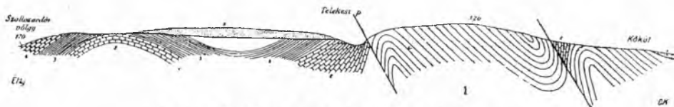
6. ábra. Szelvény a rudabányai hegységen keresztül.
