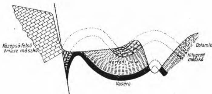
5. ábra. Egyik martonyi-i vasérckutatás szelvénye.
