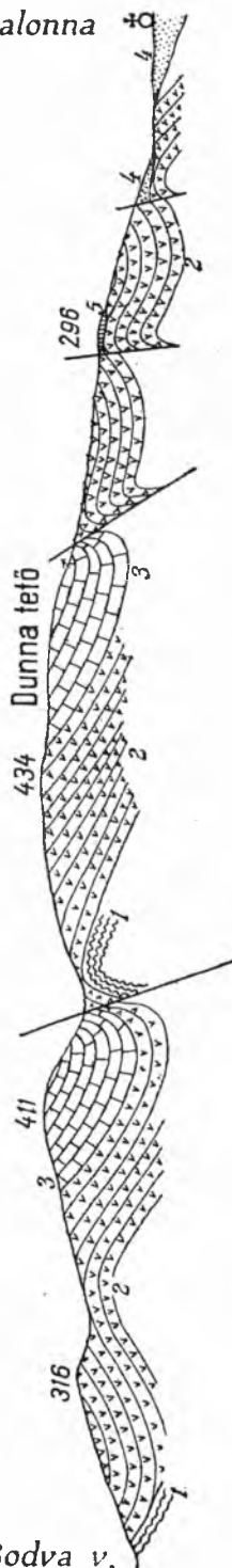
7. ábra. Szelvény a hegység északibb részén át, Szalonnától északnyugati irányban. 1 = werfeni rétegek, 2 = középsőtriász dolomit, 3 = középső- felsőtriász mészkő, 4 = pliocén képződmények, 5 = pliocén forrásmész-kő.
