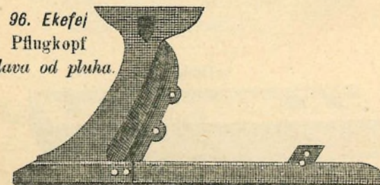
97. Eketalp Pflugsohle Podessva.
