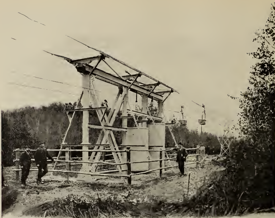
RÉSZLET A „CONCORDIA“ VASGYÁR BÁNYATÁRSULAT SODRONYPÁLYÁJÁBÓL.
