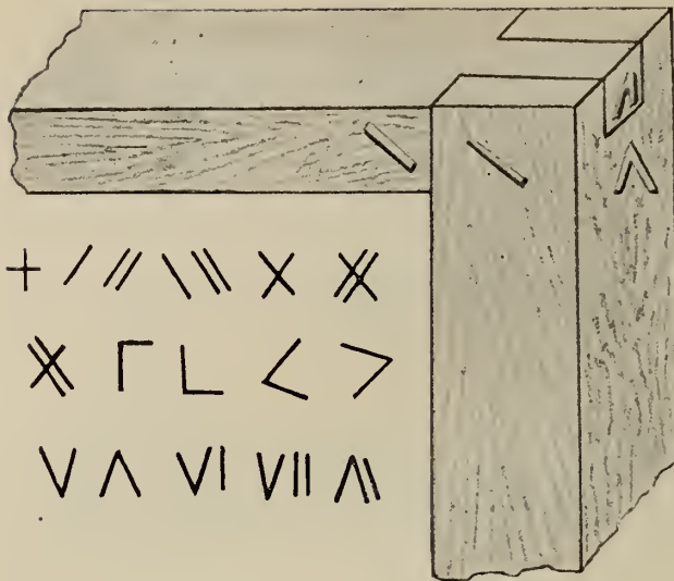
ÁCSJEGYEK A BARKÓSÁGON.
