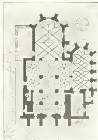
V. SZEPESVÁRALJAI SZERKESZGÉNY ALAPRAJZA.
