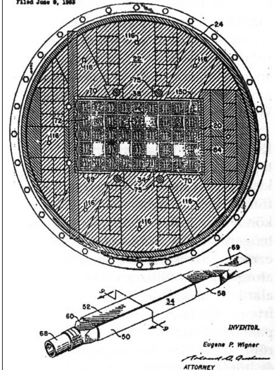
Wigner Jenő egyik reaktorszabadalma
