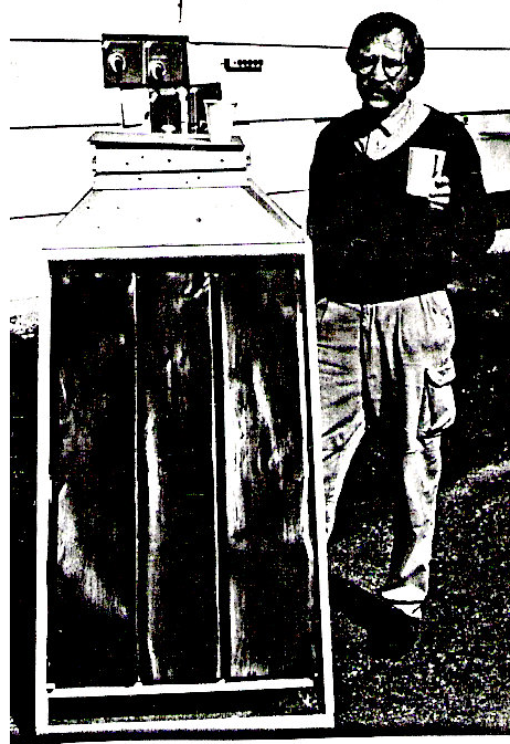
Ausztriában, 1994-ben épült hordozható szolár szárító (a szerző építése)
