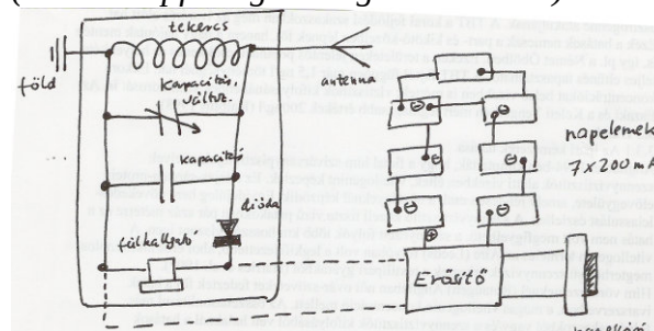
Szolar rádió, gemkapcsokból
