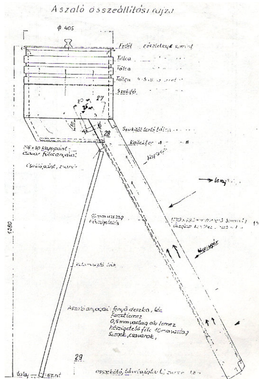
A kis szolár szárító rajza
