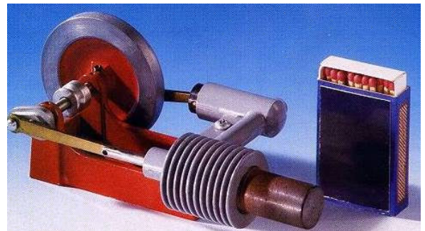
Hőlégmotor, 110 EUR, www.stirlingmotor.com
