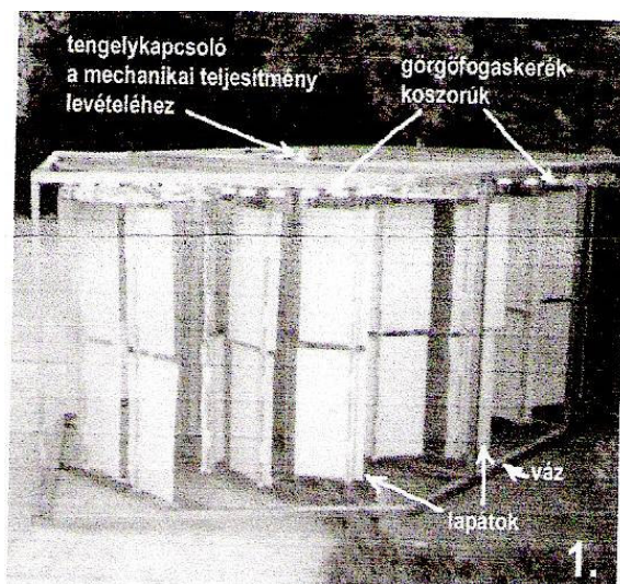
Vízáram-motor, Salca János, Bp.
