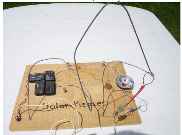
Szolár necsipogj-játék: a karikát áthúzni
