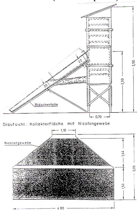
Szárító torony, Nicolon fóliával (bajor)
