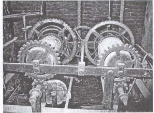
A toronyóra szerkezete
