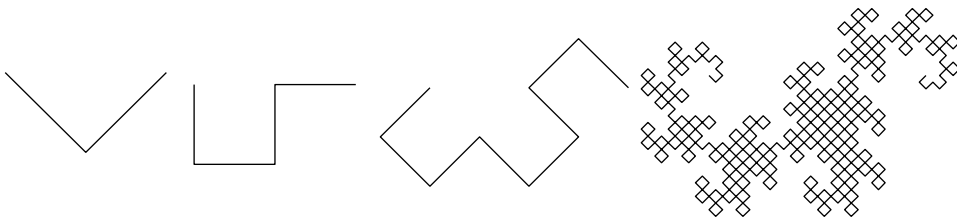
sárkány 90 1 1
