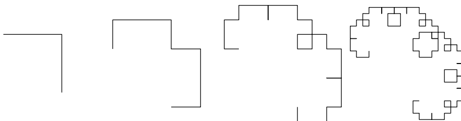
Levy 250 1
