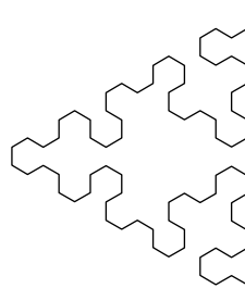
nyílhegy 5 0 4
