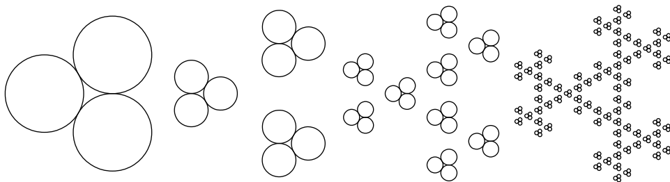
körök 502
