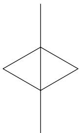
Peano_Koch 5 0 2
