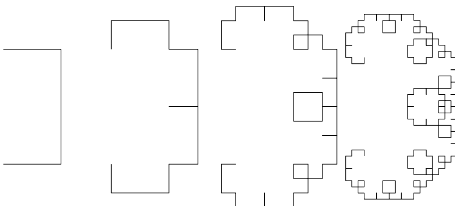
Levy1 100 1
