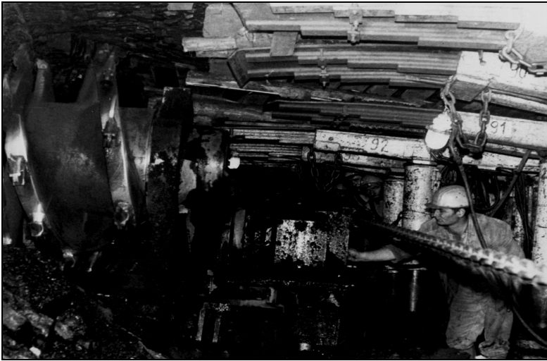
Fletcher önjáró biztosító egységes frontfejtés, Eickhoff-maróhengerrel
