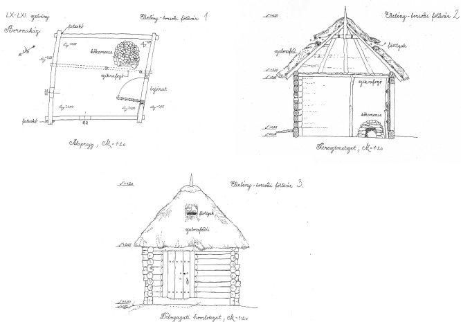
7. kép: Boronaház rekonstrukciós rajza.
