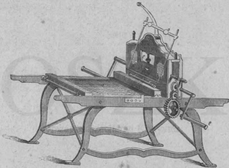
Vas könyomású sajtó.
