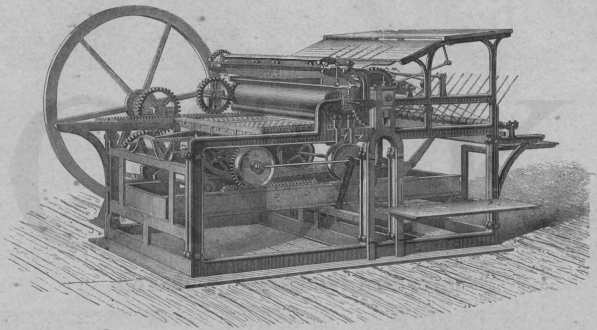
König és Bauer egyszerű gyorsajtója vasuti mozgással és önrakóval.
