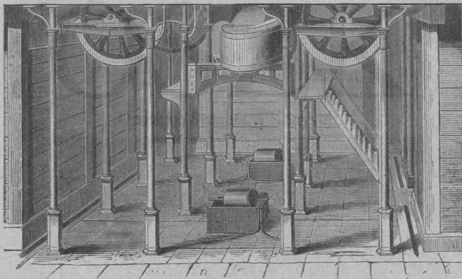
Hollandi terem a papirosgyárban.
