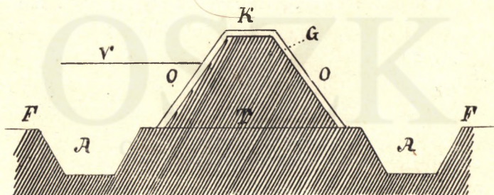
13. Gátépítés. T. a gát talpa; K. a gát koronája, O. O. a gát oldala vagy lejtője; G. gyepelés; A. A. árkolás a gát mentén; F. tőfenék; V. a víz színvonala.
