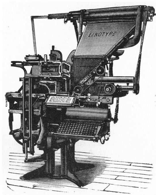
4. ábra. Linotype sorszedő-, öntő- és osztógép.
