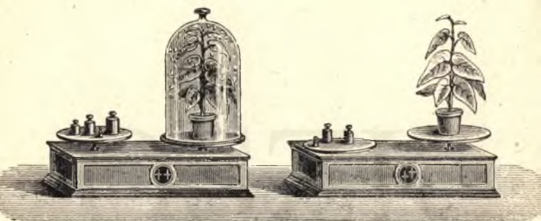
9. kép. A növényből elpárolgó víz mérése mérleggel.
