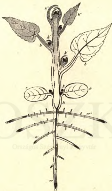
8. kép. A növény hosszanti metszete , amelyben a fekete vonalak a vízszállító pályák (edénnyalábok) futását jelzik.
