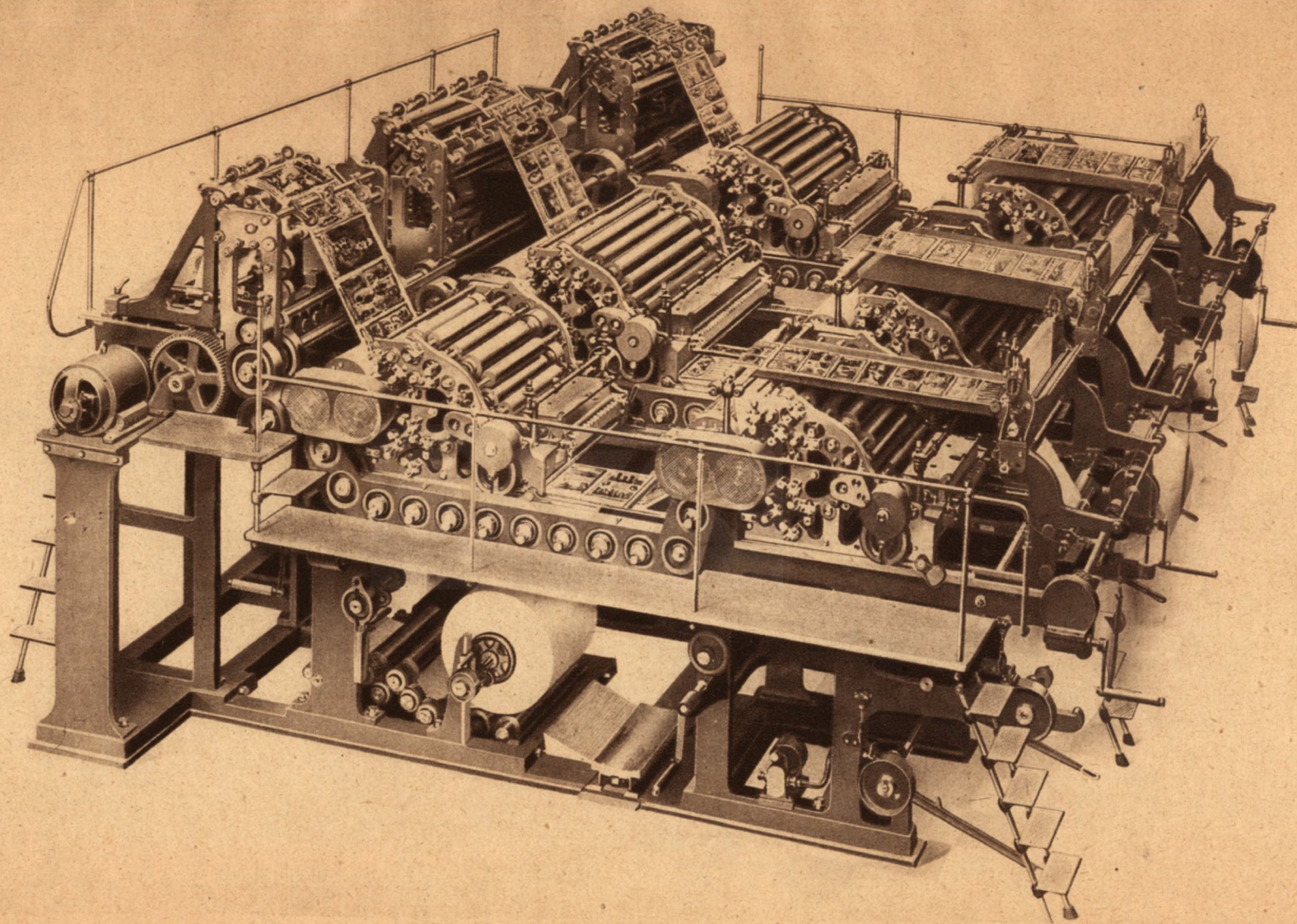
Három körforgógép (rotációs) egybeépítve. Ez a gépcsoport 80 oldal képesűságot nyom, vág, fűz és hajtogat egyszerre és ezzel a munkamenettel 16 rendes újságnymógép és 40 ember munkáját végzi el. A rotációsgépterem az utcai alagsorban van. Az első teremben levő 5 illusztrációs körforgógép éjjel-nappali üzemben naponta 20 tonna papírt tud feldolgozni.
