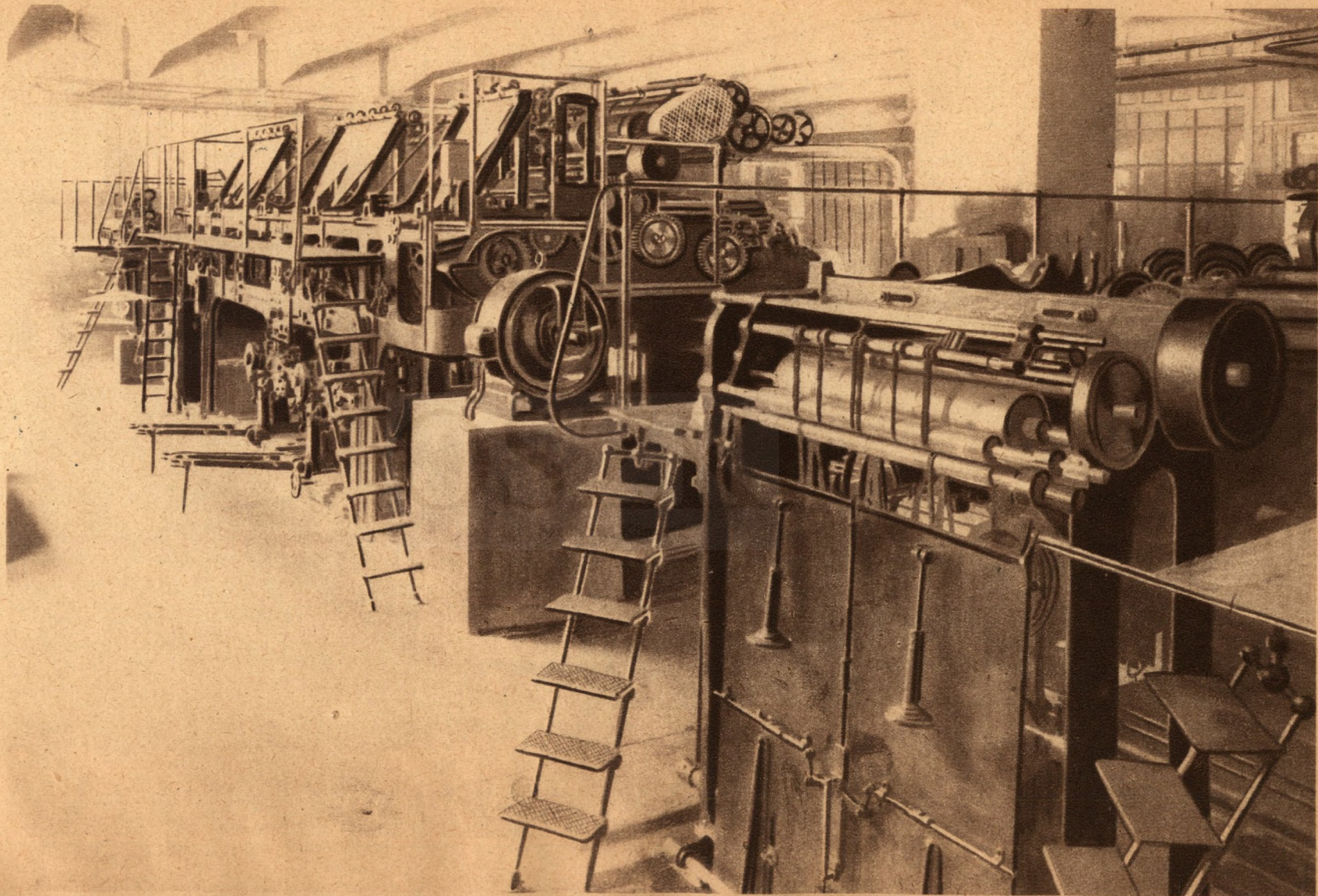
Tolnai Nyomdai Műintézet és Kiadóvállalat R.-T. Rotációs gépterem. Képünk öt illusztrációs rotációs gépet mutat be, mely az utcai alagsorban van elhelyezve. E gépek papirfogyasztása éjjel-nappali üzem mellett, napi két waggon.
