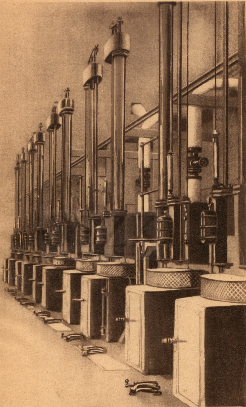
A fűtőház, melyben egy gőzfejlesztő-készülék is van, a rotációs gépekben szaladó papiros nedvesítésére.
