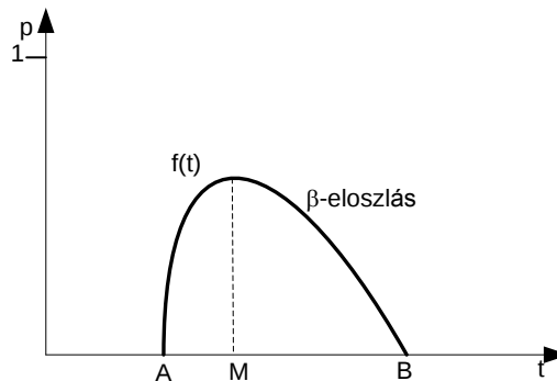
1.3.5-1 ábra: a \beta -eloszlás sűrűségfüggvénye
