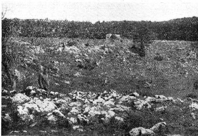
9. ábra. Dolina a Képeskúti akol körül. Atmérője k. b. 30 m. Hátterben az erdő előtt eseh határerőd látszik.
