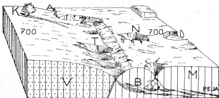
11. ábra. Képeskúti akol környékének tömörszelvénye. — A. Barlangnyílás. — B. Barlang. — D. Dolina (9. fénykép). — K. Képeskúti akol. Összehasonlító mérték az iderajzolt fa. — M. Mészkő. — N. Víznyelő (10. fénykép). — T. Rendellenes alakú víznyelők a tektonikus vonalakon. — V. Werfeni pala. — Z. Betömődött víznyelő.
