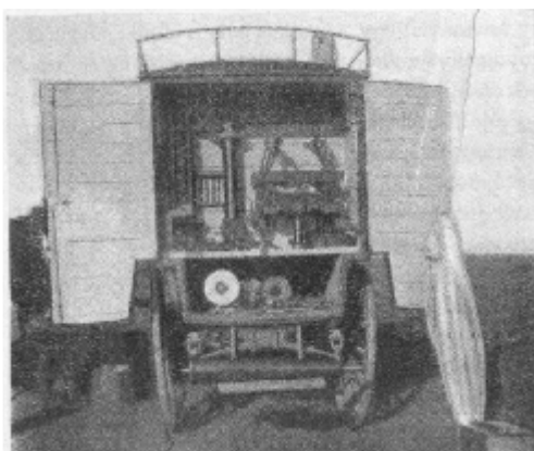
Eötvös által tervezett műszerkocsi és mérősátor
