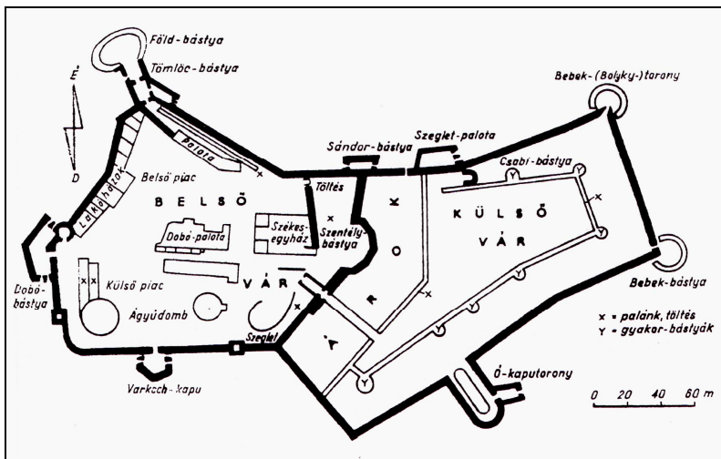
8. kép. Az egeri vár alaprajza az 1552. évi ostrom idején (SUGÁR István, 1984. 4. kép.)
